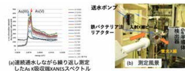
図7.SPring8における連続通水条件下でのXAFS測定による砒素除去機構解明
