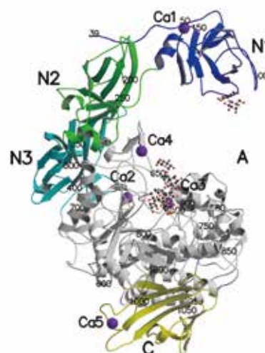
微生物プルラーゼの構造 5個のドメインから成る。
