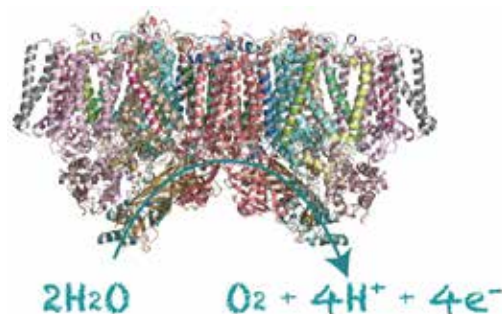
光化学系IIのタンパク質立体構造
