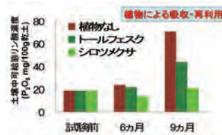
図6. 家畜排せつ物消化液の投与試験 可給態リンと植物成長の関係、エストロゲンの植物濃縮係数
