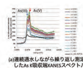
図7. SPring8における連続通水条件下でのXAFS測定による砒素除去機構解明
