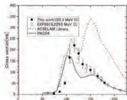
図1. 重イオン等の入射による放射化断面積測定の様子と測定結果
