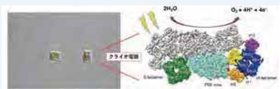
ツノケイソウ( Chaetoceros gracilis )の顕微鏡写真(左)と、その光化学系II - 集光性色素タンパク質複合体の構造(右)
